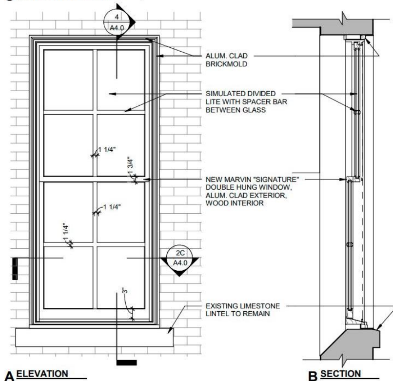
A ELEVATION
