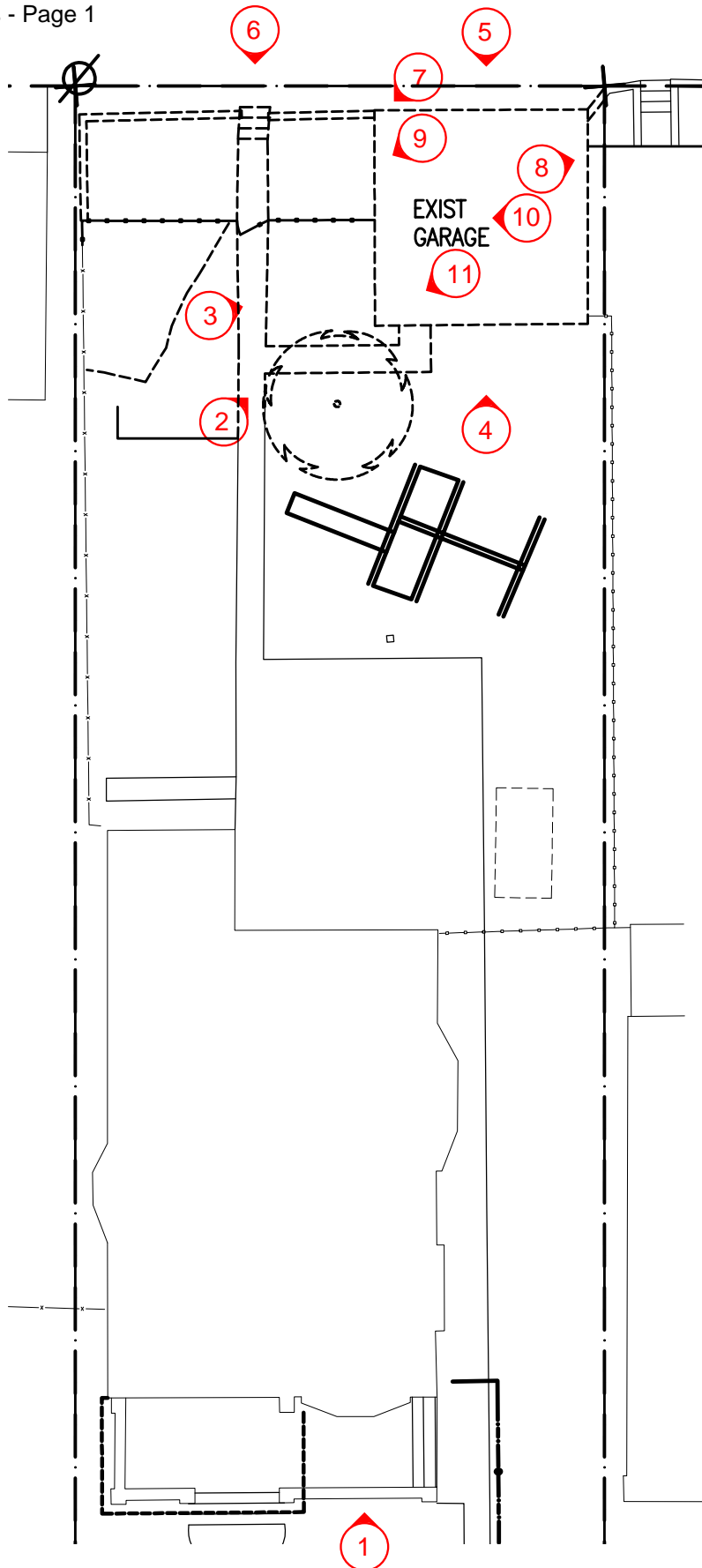
1 EXISTING SITE PLAN SCALE: N.T.S.
