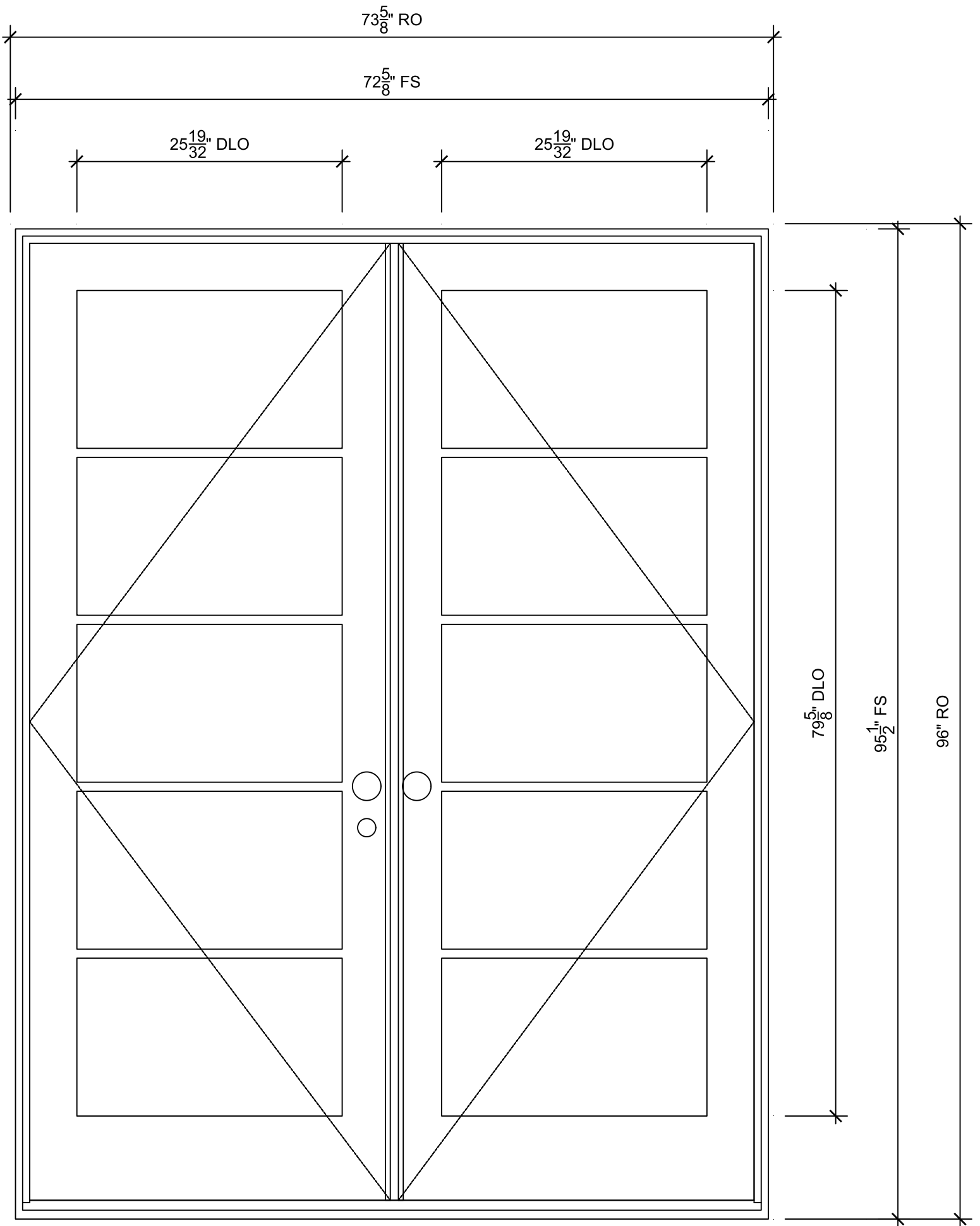
6080 XX DOOR
