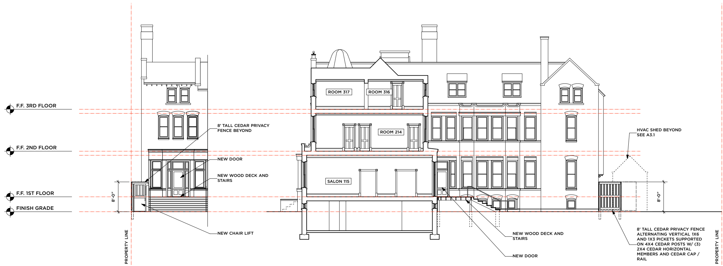
2 PARTIAL ELEVATION A3.3 SCALE: 1/8" = 1' - 0"
