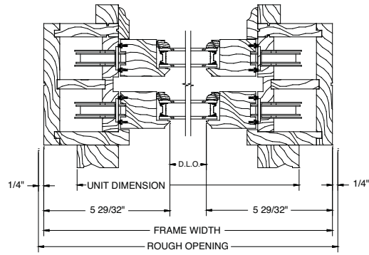
JAMB
