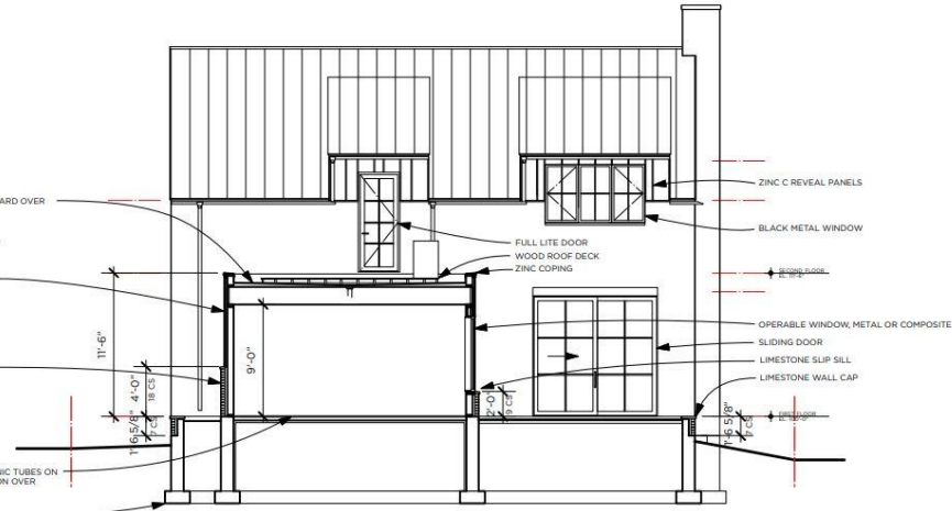
1 CONNEX SECTION A3.2 SCALE: 1/8" = 1'-0"
