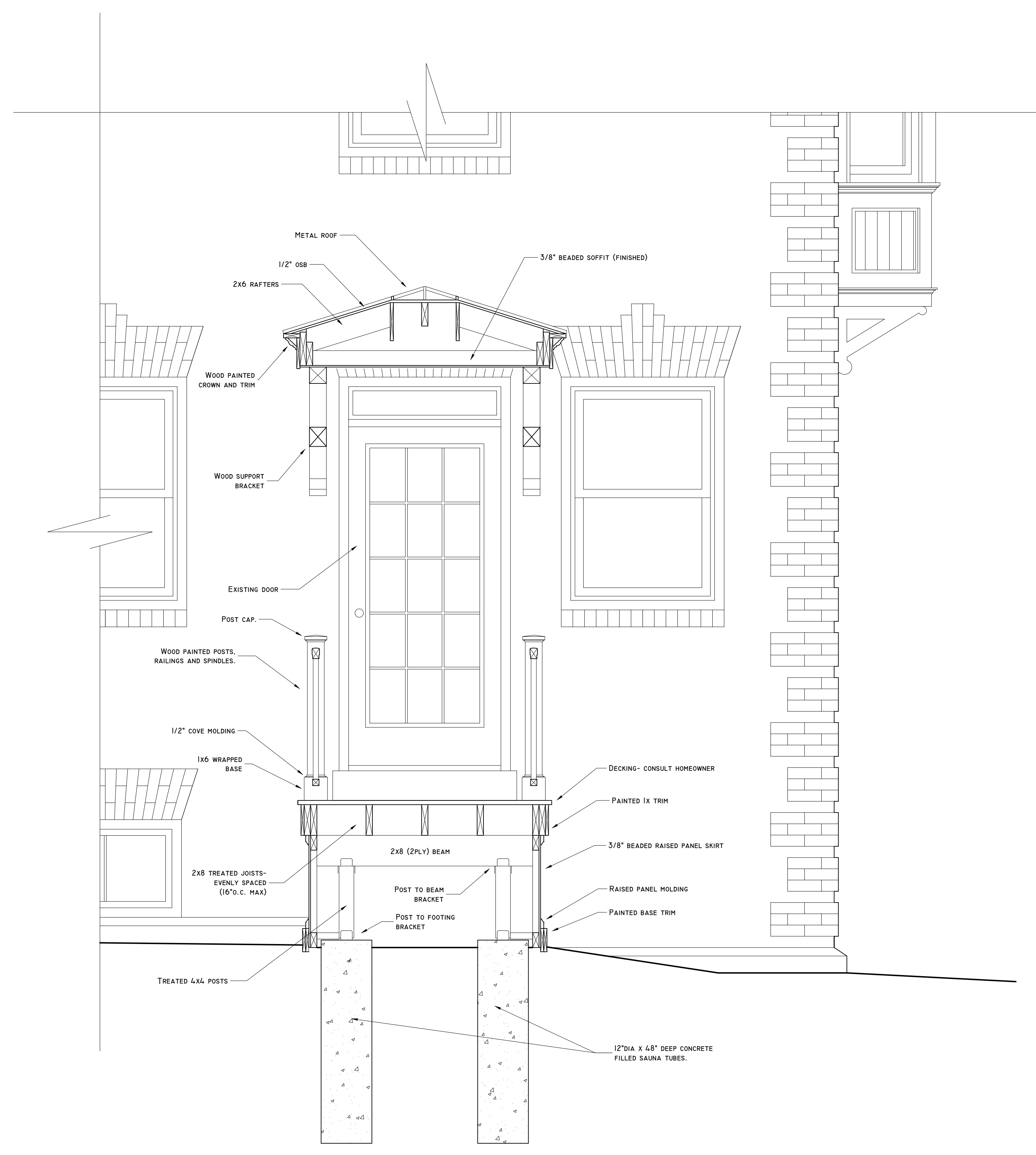
SECTION A SCALE: 3/4" = 1'0"
