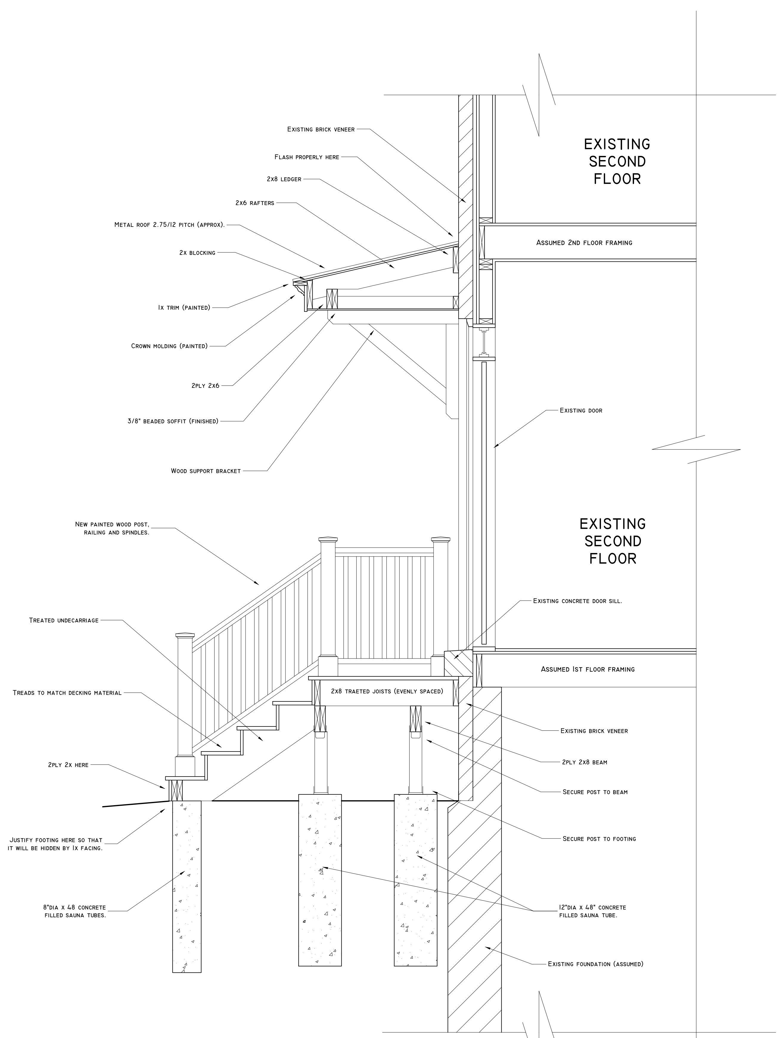
SECTION B SCALE: 3/4" = 1'0"
