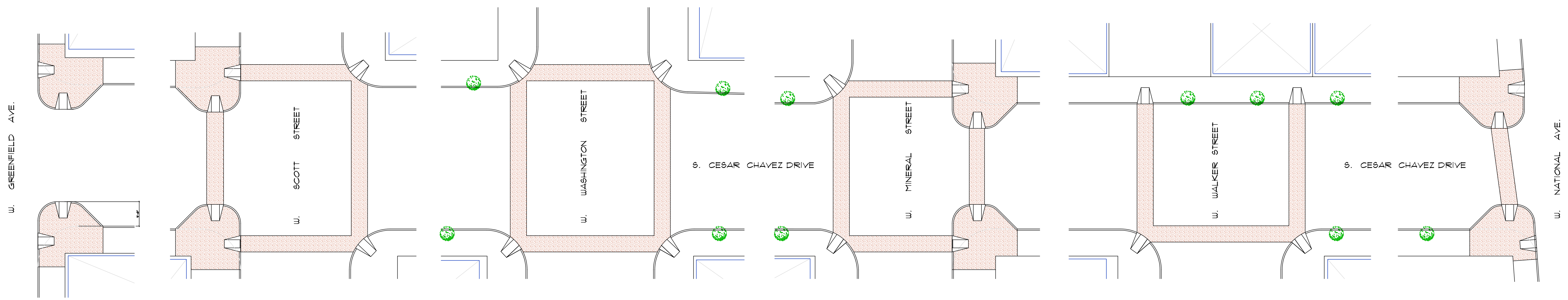
2 NEW CROSS WALKS A-1 Scale: 1/16"=1'-0"
