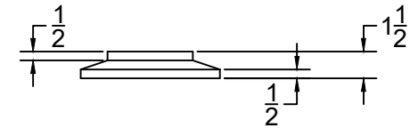
COLUMN CAP
