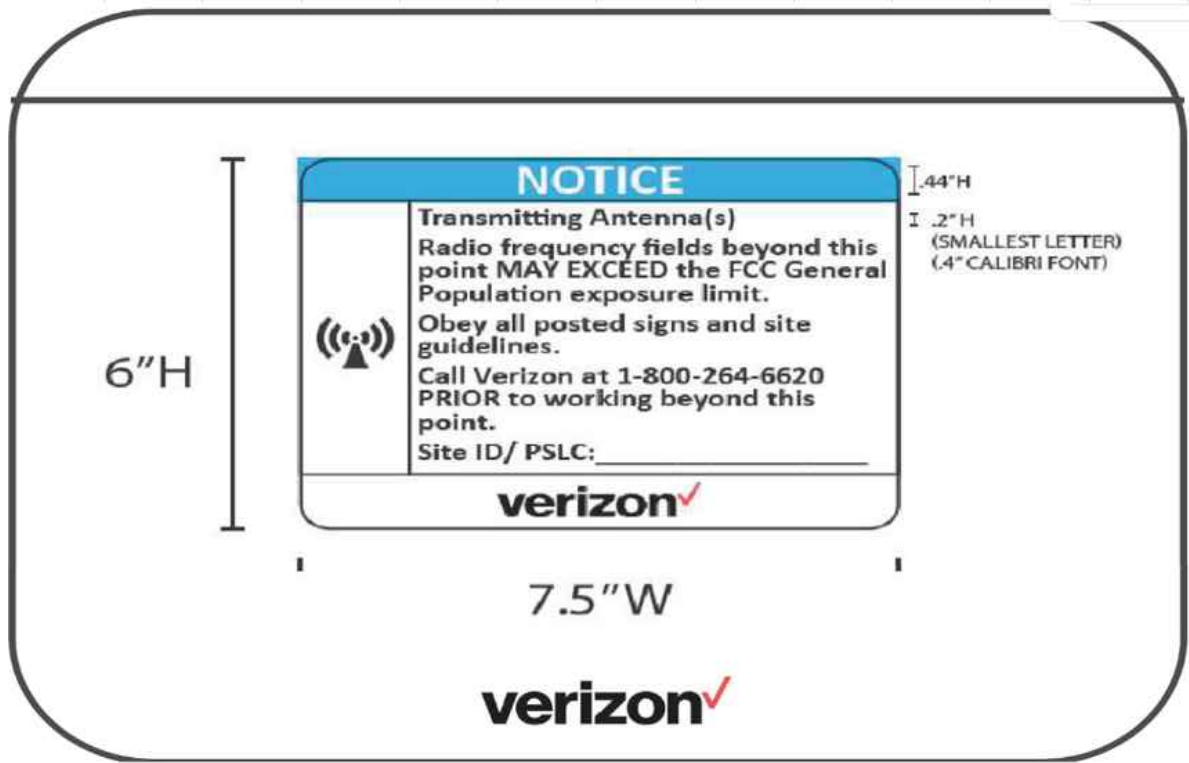
2 REQUIRED SIGNAGE SCALE: N.T.S.
